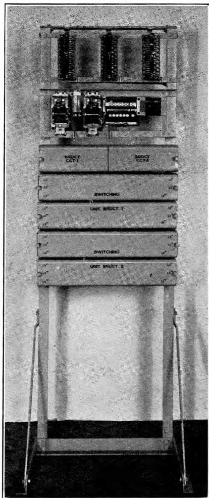
FIG. 2.—SWITCHING UNIT.
