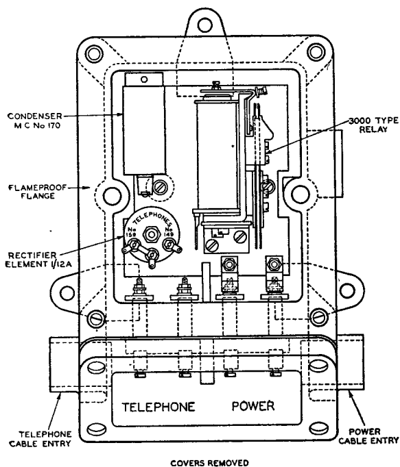
FIG. 6.—RELAY UNIT.
